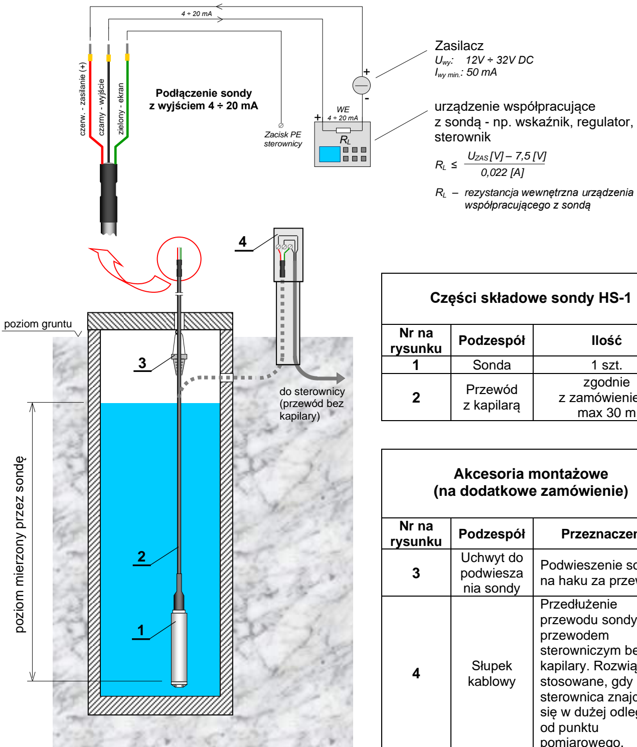
Rys.1 Montaż sondy HS-1 w zbiorniku
